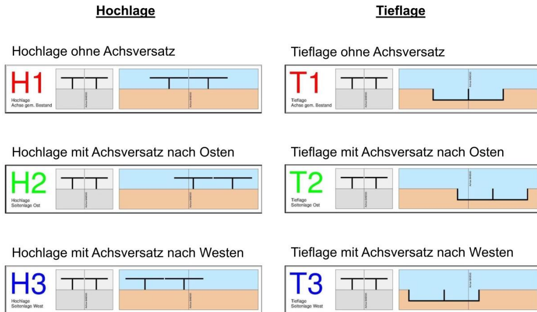
Abbildung 3.18 Variantenübersicht der Hauptvarianten in Hoch- und Tiefloge
