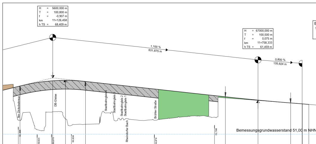
Abbildung 3.34 H1T1b – Höhenplanarstellung nördlicher Abschnitt
